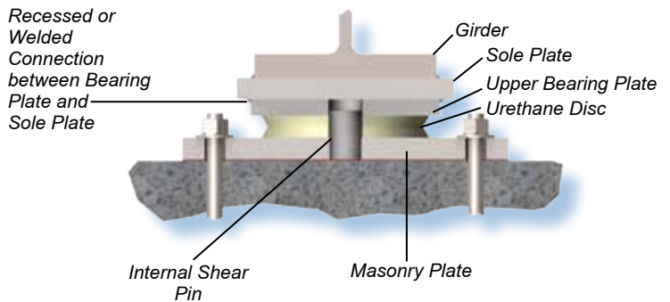
3-Plate Design
